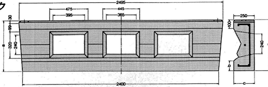
■寸法表(3分勾配)
