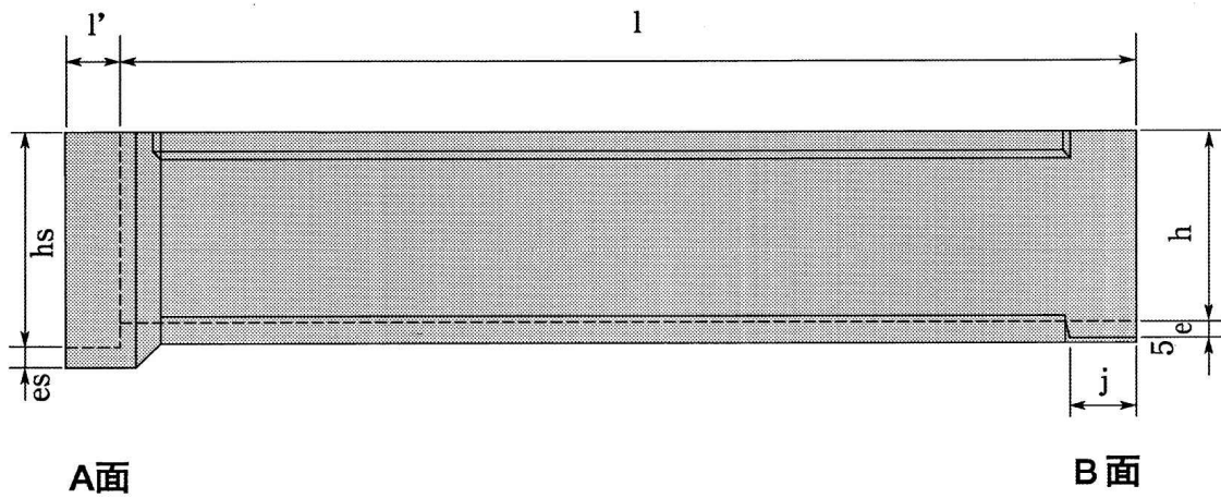
(側面図)
